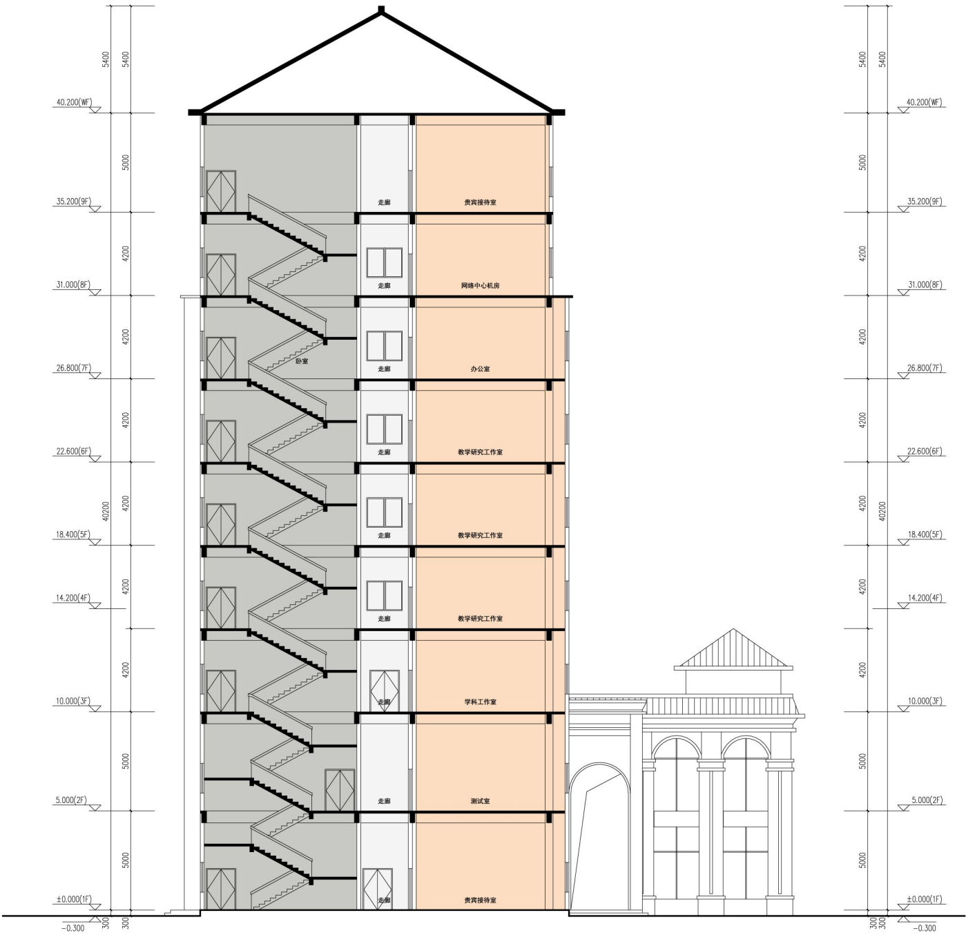
学术综合楼 1-1剖面图
