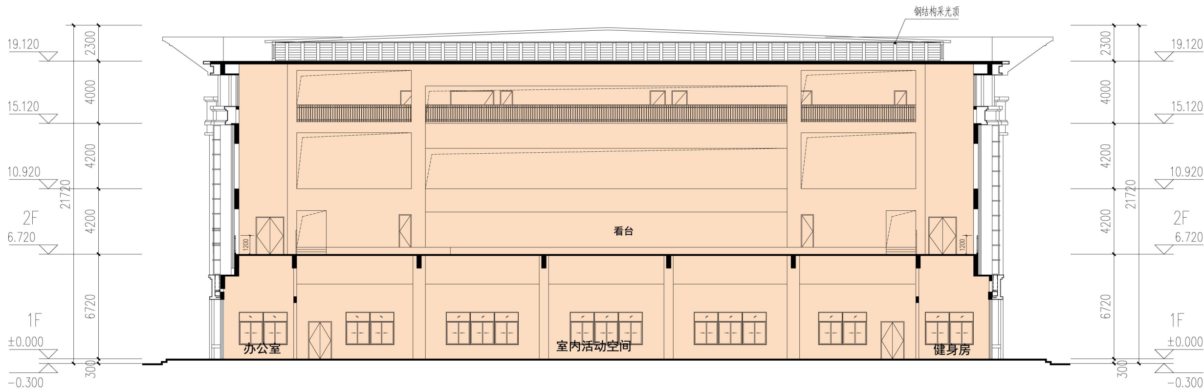
体育馆剖面图
