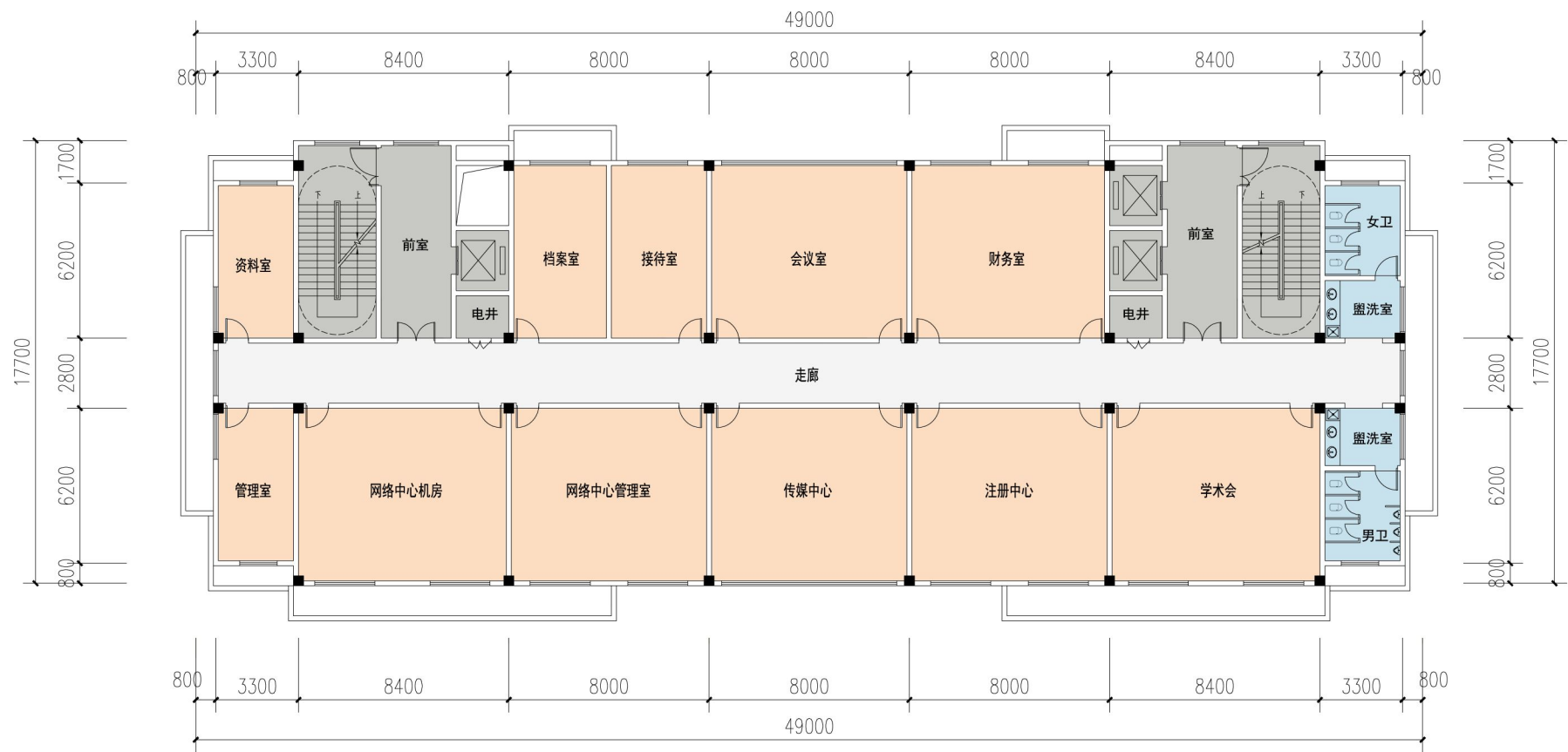
学术综合楼 八层平面图
