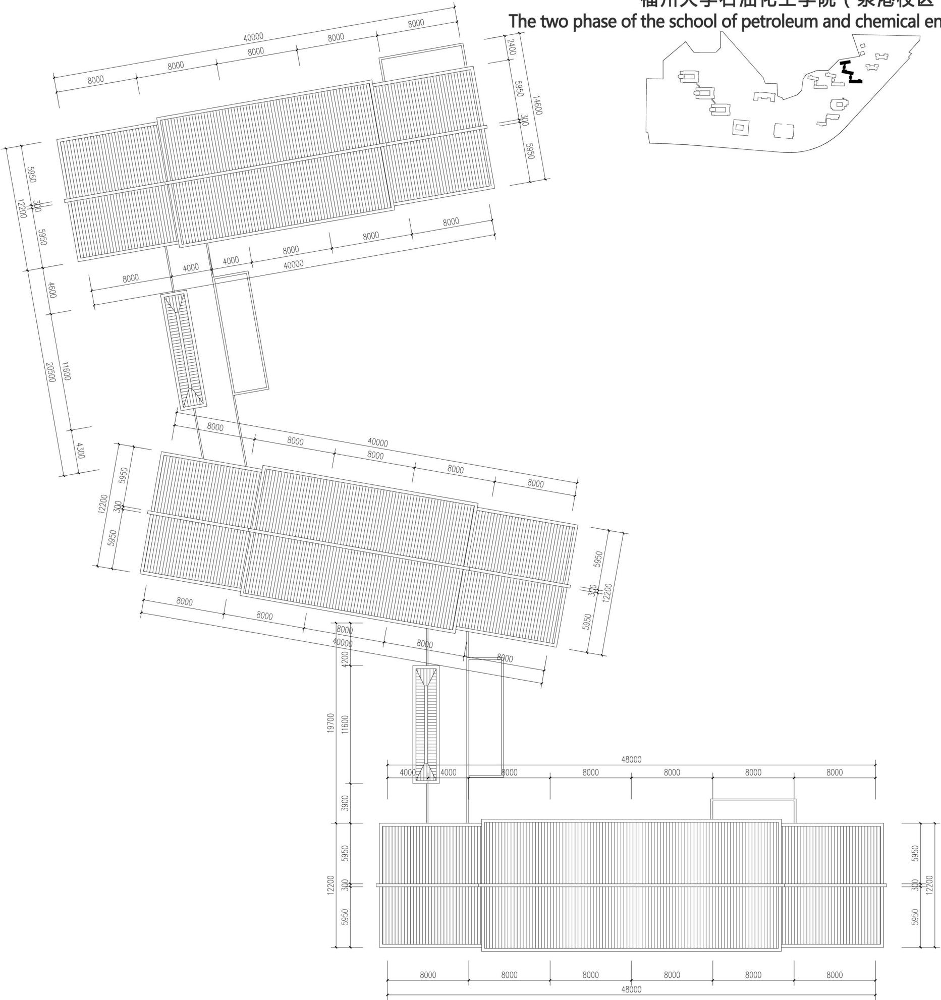
学生公寓 屋面平面图
