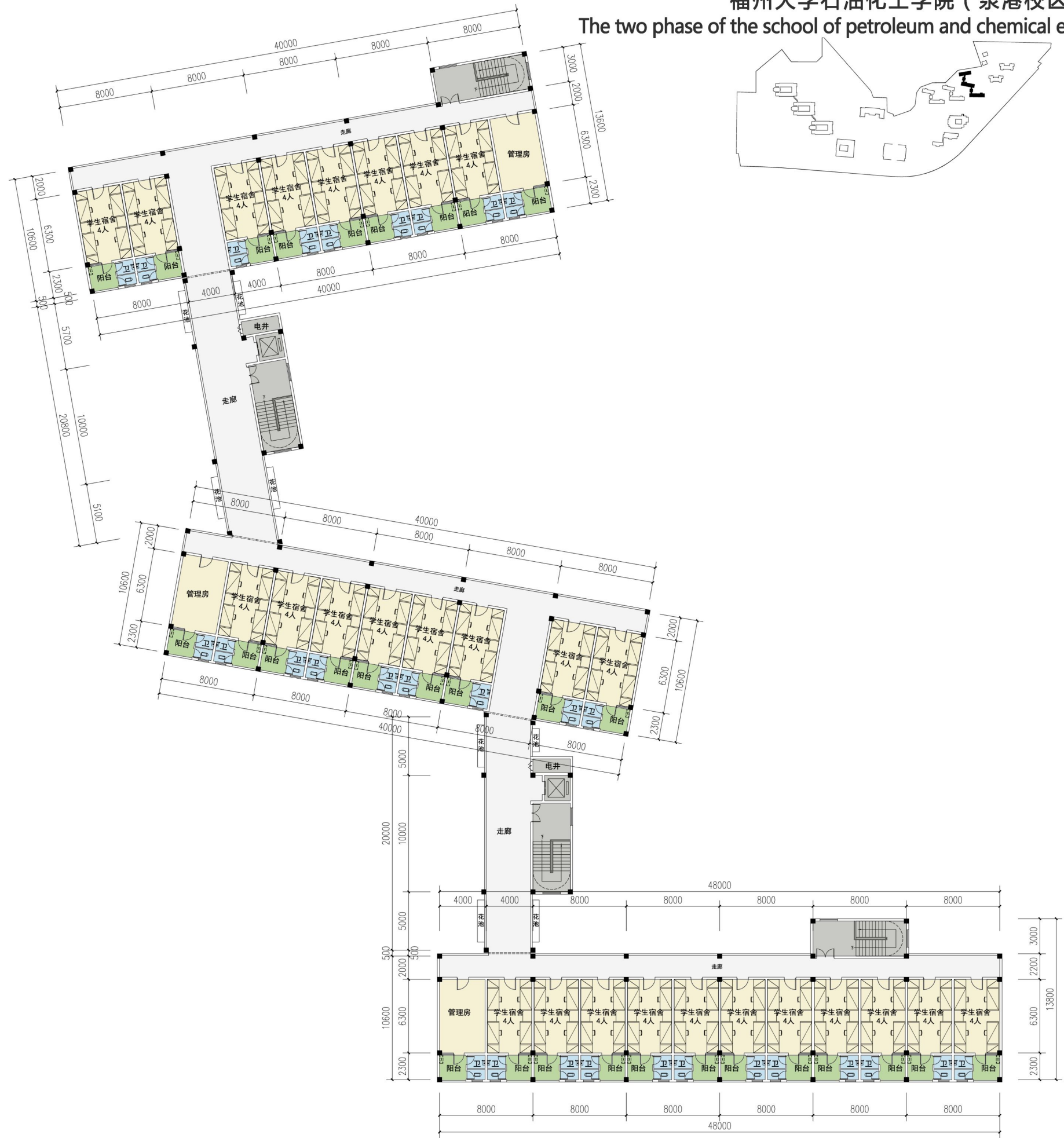
学生公寓 七层平面图 19.600
