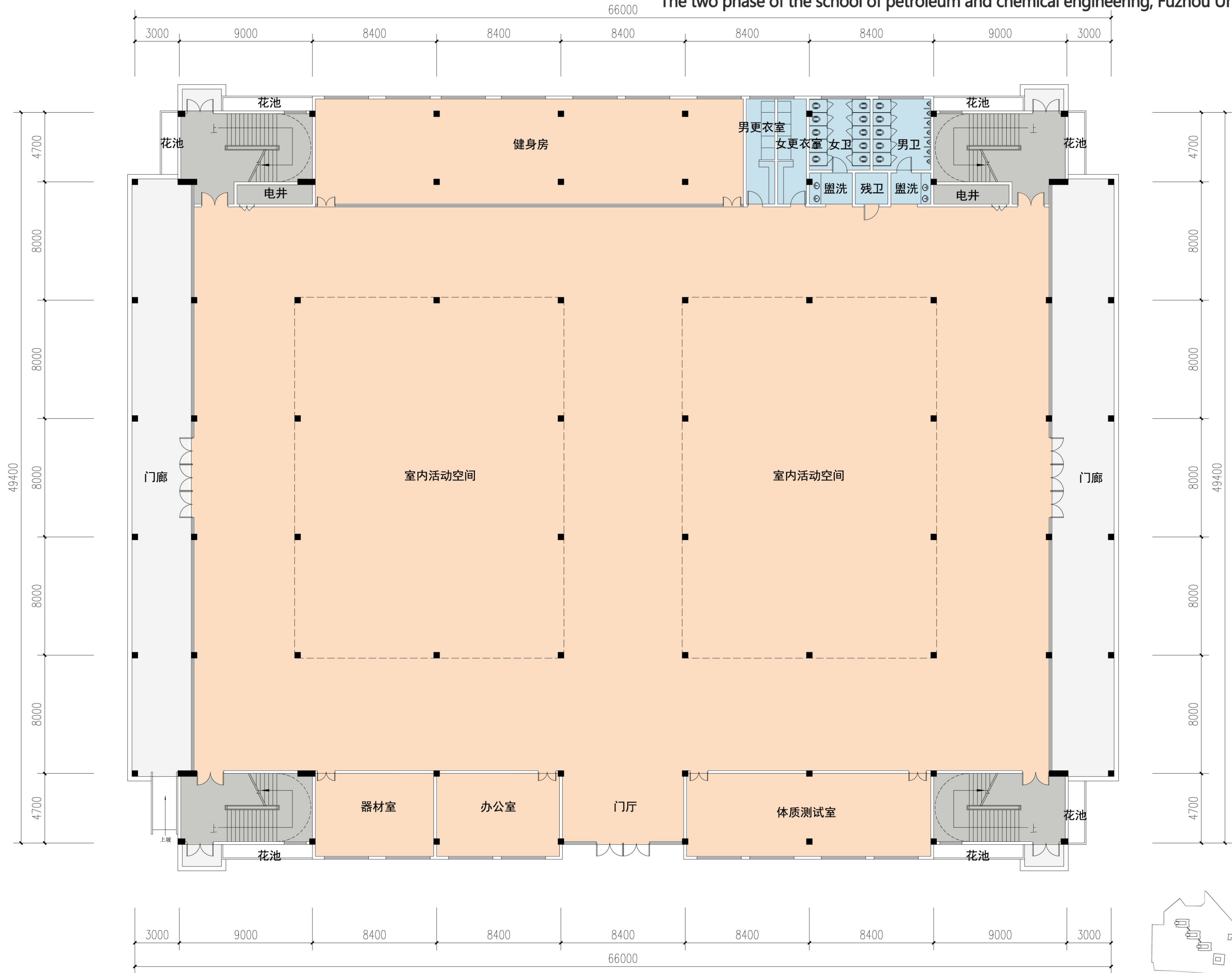
体育馆一层平面图
