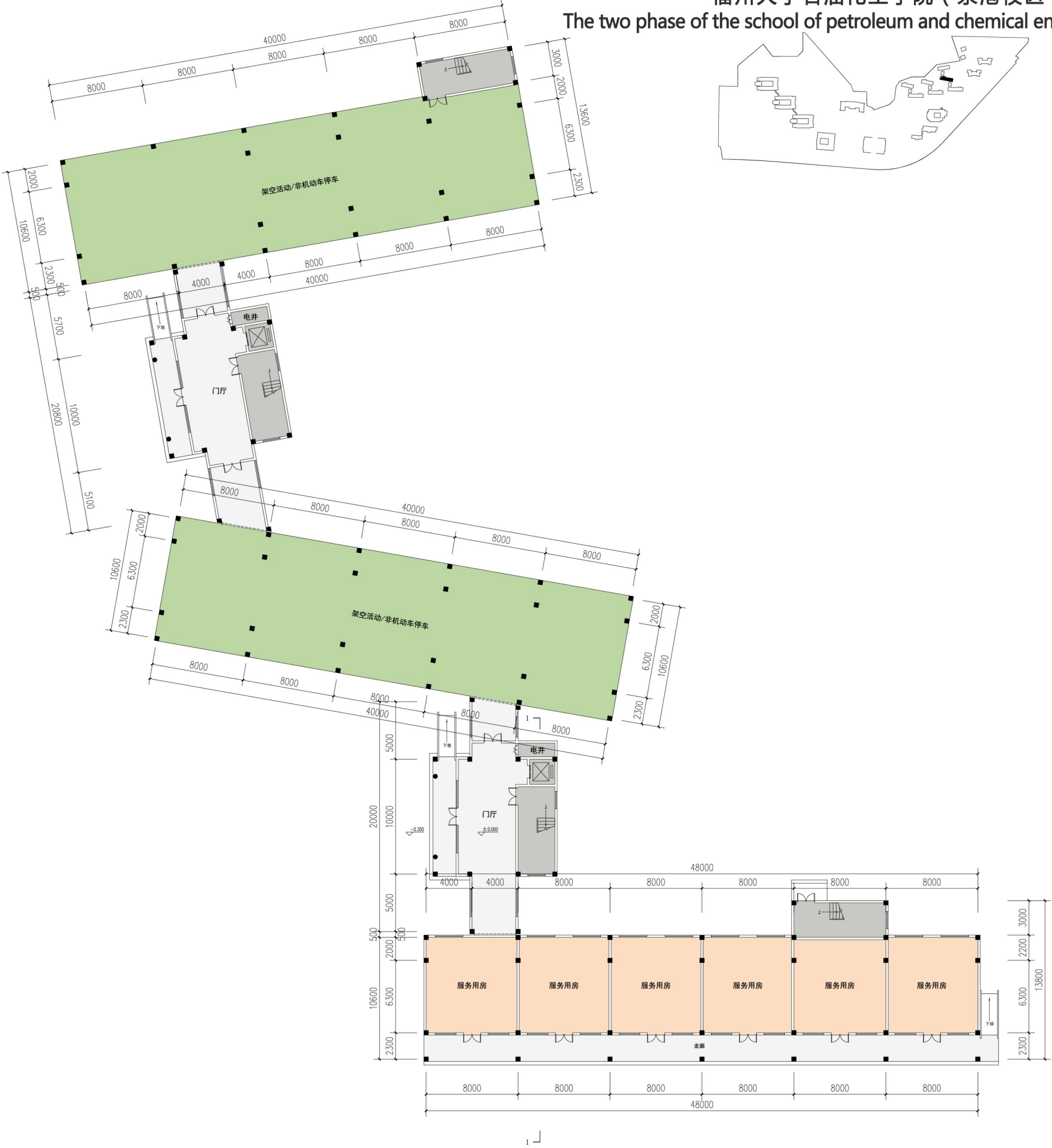
学生公寓 一层平面图
