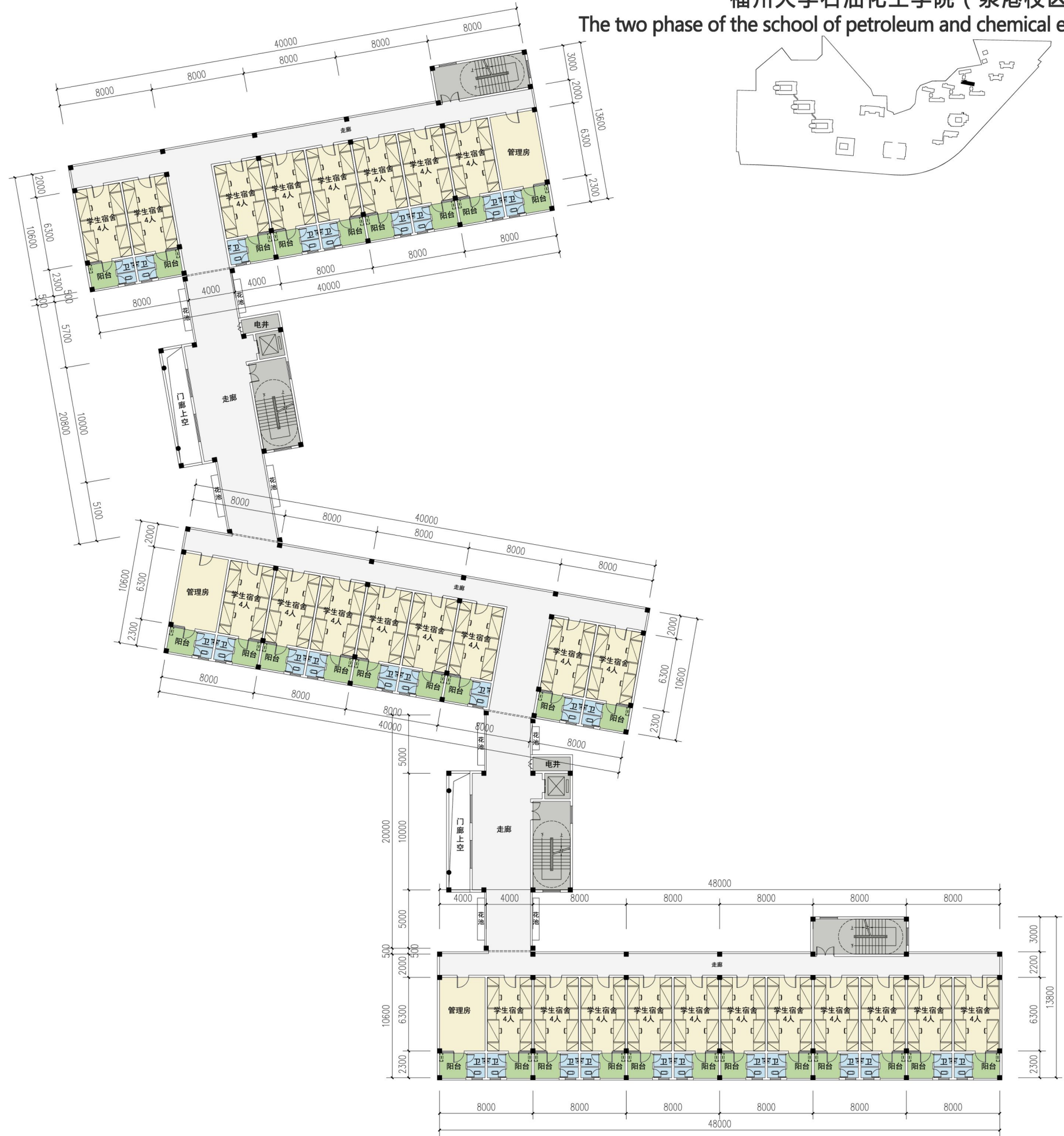
学生公寓 二层平面图
