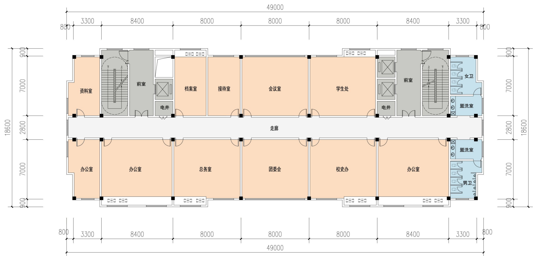
学术综合楼 七层平面图
