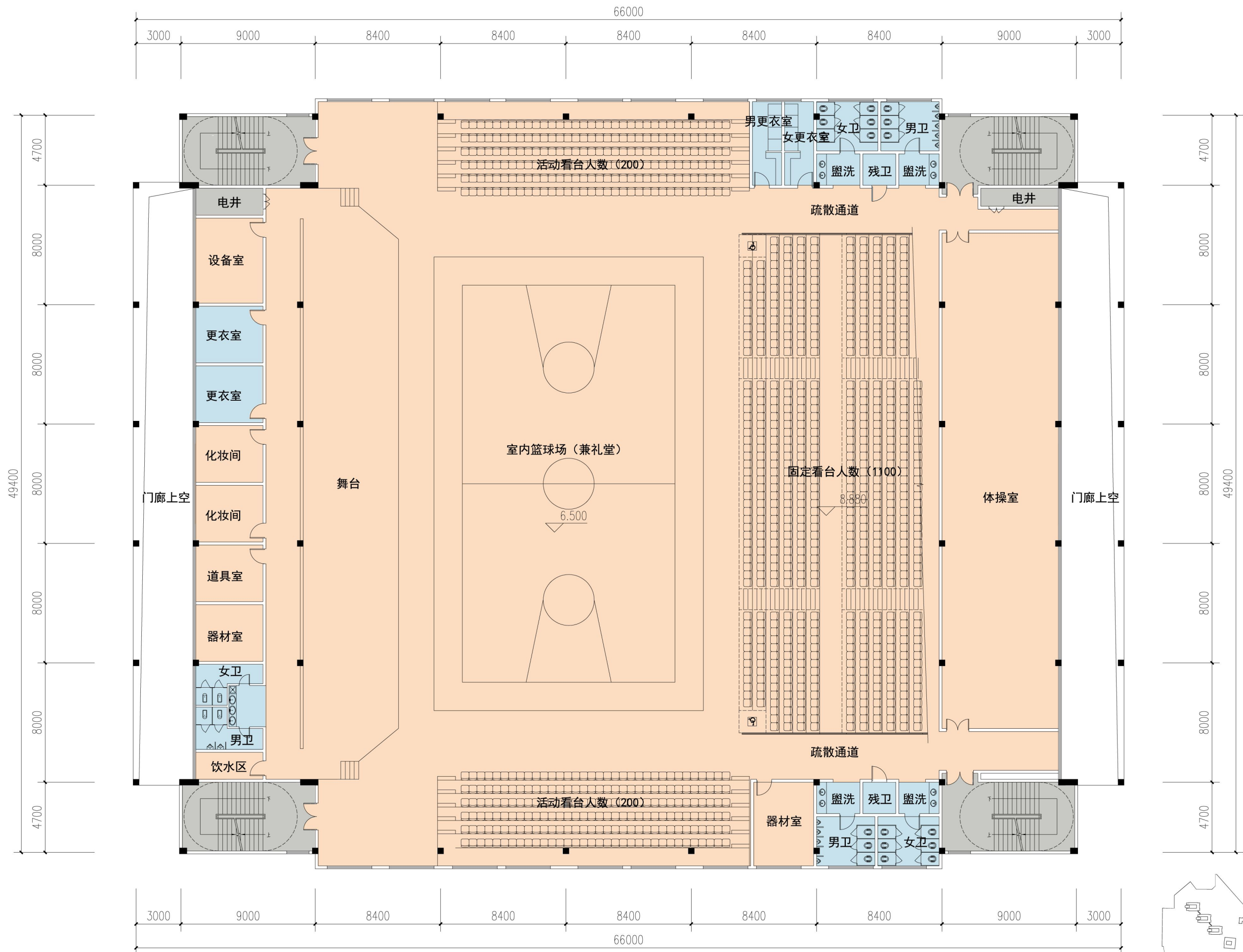
体育馆二层平面图
