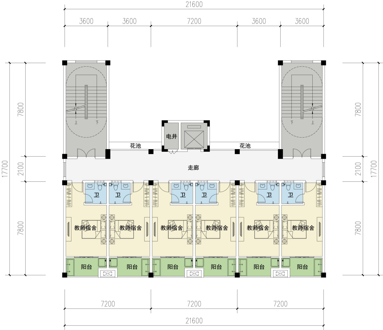
教师公寓 九层平面图
