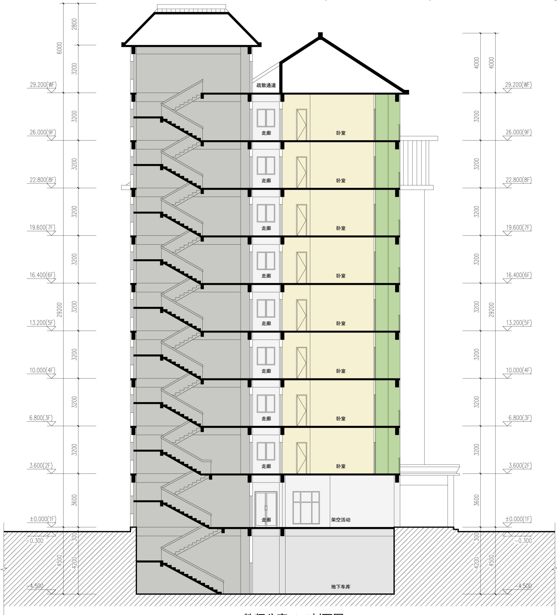
教师公寓 1-1剖面图
