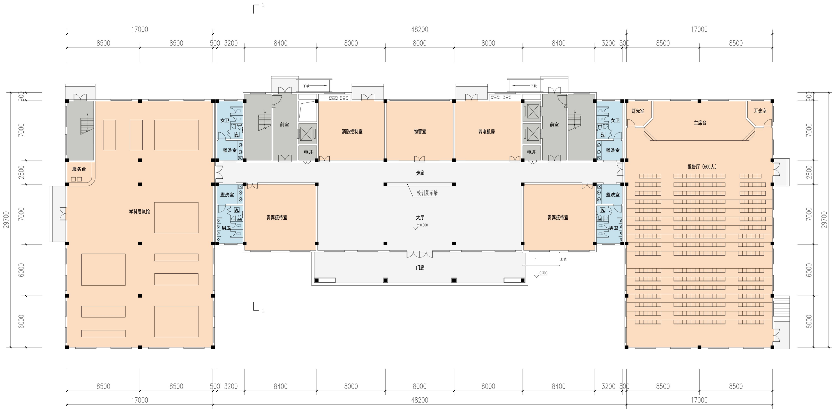
学术综合楼 一层平面图
